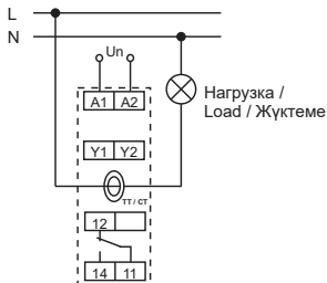
а) без трансформатора тока / without current transformer / ток трансформаторыныңсыз
