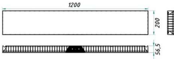
Рисунок 1 Светильник «L-school 55 Premium/Em»
