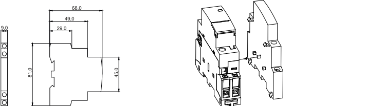
Рисунок 2 – Габаритные размеры контакта дополнительного / Figure 2 – Overall dimensions of auxiliary contact
