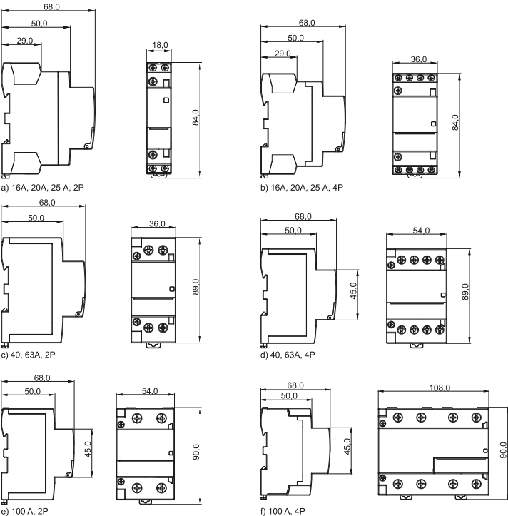
Рисунок 1 – Габаритные размеры контакторов / Figure 1 – Overall dimensions of contactors
