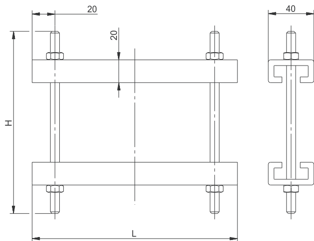
Рисунок / Figure 1 – Прижим крышки лотка усиленный / Reinforced hold-down clamp for cable tray cover
