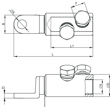
Рисунок 1 – Наконечники до 1кВ / Figure 1 – Lugs up to 1kV / 1 сурет – 1 кВ-ге дейінгі ұштықтар
