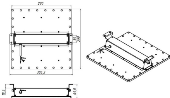
Рисунок 1 Светильник «L-parking».
