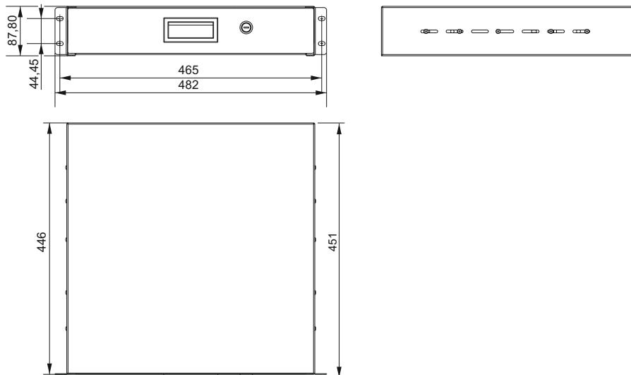
Рисунок 1 – Внешний вид ящика / Figure 1 – Appearance of the drawer / 1-сурет – Жәшіктің сыртқы көрінісі
