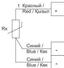
б) 3-проводная / b) 3-wire / б) 3 сымды
