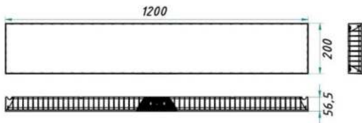
Рисунок 1 Светильник «L-school 32 S Premium/Em»
