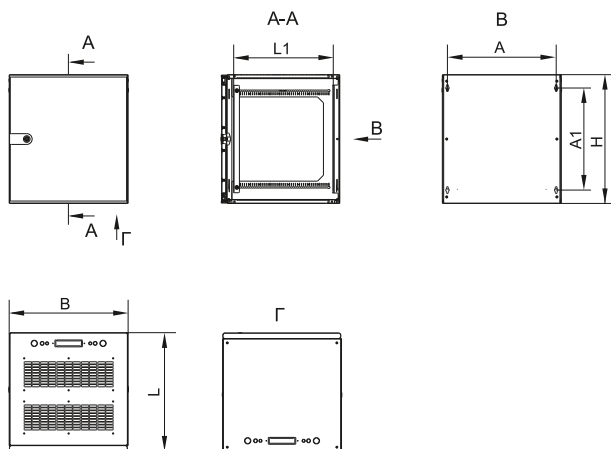
Рисунок 1 – Внешний вид шкафа / Figure 1 – Appearance of the cabinet / 1 сурет – Шкафтың сыртқы көрінісі
