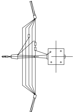
Схема отведения к входу в здания в одну сторону 2х жил СИП
