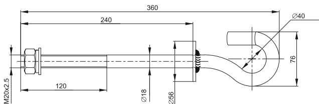
Рисунок 2 – Внешний вид и габаритные размеры крюка монтажного В 20/240 / Figure 2 – Appearance and overall dimensions of mounting hook В 20/240 / 2 сурет – 20/240 В монтаждай ілмегінің сыртқы көрінісі және габариттік өлшемдері
