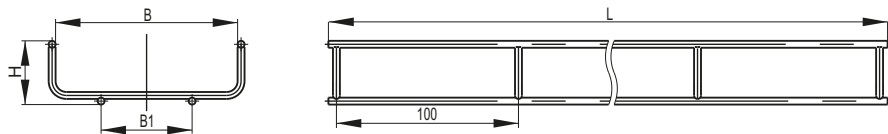
Рисунок 1 – Лотки высотой H = 35, 50 мм / Figure 1 – Trays with height H = 35, 50 мм / 1 сурет – Биіктігі H = 35, 50 мм науалар
