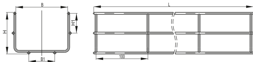
Рисунок 2 – Лотки высотой H = 80, 100 мм / Figure 2 – Trays with height H = 80, 100 мм / 2 сурет – Биіктігі H = 80, 100 мм науалар
