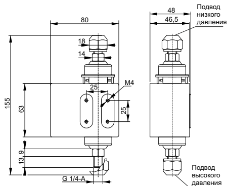
Рисунок 1 – Габаритные и установочные размеры реле
