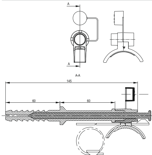
Рисунок 1 – Габаритные и установочные размеры комплекта / Figure 1 – Overall and mounting dimensions of the kit / 1 сурет – Жиынтықтың габариттік және орнату өлшемдері
