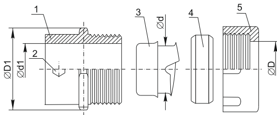
1 - корпус; 2 – болт (винт); 3 - оконцеватель МК; 4 - уплотнитель; 5 - накидная гайка.
