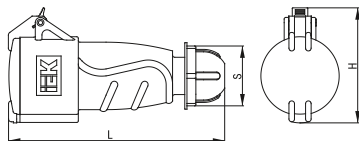
Рисунок 4 – Габаритные размеры соединителей типа ССИ-213, ССИ-214, ССИ-215, ССИ-223, ССИ-224, ССИ-225 / Figure 4 – Overall dimensions of plug and socket-outlets SSI-213, SSI-214, SSI-215, SSI-223, SSI-224, SSI-225 / Сурет 4 – СИ-213, ССИ-214, ССИ-215, ССИ-223, ССИ-224, ССИ-225 типті жалғастырғыштардың габариттік өлшемдері
