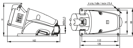
Рисунок 6 – Габаритные размеры соединителей типа ССИ-113, ССИ-114, ССИ-115 / Figure 6 – Overall dimensions of plug and socket-outlets SSI-113, SSI-114, SSI-115 / Сурет 6 – ССИ-113, ССИ-114, ССИ-115 типті жалғастырғыштардың габариттік өлшемдері
