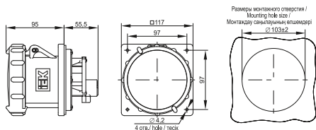
Рисунок 12 – Габаритные размеры соединителей типа ССИ-433, ССИ-434, ССИ-435 / Figure 12 – Overall dimensions of plug and socket-outlets SSI-433, SSI-434, SSI-435 / Сурет 12 – ССИ-433, ССИ-434, ССИ-435 типті жалғастырғыштардың габариттік өлшемдері
