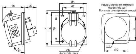
Рисунок 11 – Габаритные размеры соединителей типа ССИ-423, ССИ-424, ССИ-425 / Figure 11 – Overall dimensions of plug and socket-outlets SSI-423, SSI-424, SSI-425 / Сурет 11 – ССИ-423, ССИ-424, ССИ-425 типті жалғастырғыштардың габариттік өлшемдері
