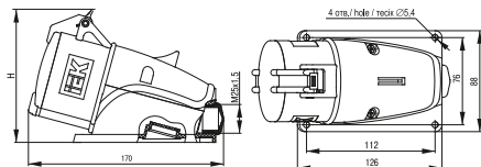
Рисунок 7 – Габаритные размеры соединителей типа ССИ-123, ССИ-124, ССИ-125 / Figure 7 – Overall dimensions of plug and socket-outlets SSI-123, SSI-124, SSI-125 / Сурет 7 – ССИ-123, ССИ-124, ССИ-125 типті жалғастырғыштардың габариттік өлшемдері
