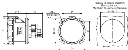
Рисунок 13 – Габаритные размеры соединителя типа ССИ-445 / Figure 13 – Overall dimensions of plug and socket-outlets SSI-445 / Сурет 13 – ССИ-445 типті жалғастырғыштардың габариттік өлшемдері
