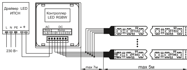
Рисунок 8 – Схема параллельного подключения многоцветной RGB, RGBW светодиодной ленты к блоку питания и контроллеру
