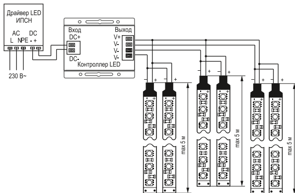
Рисунок 6 – Схема параллельного подключения к контроллеру одноцветных лент разного цвета к отдельному каналу контроллера с общим анодом
