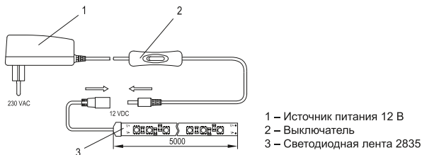
Рисунок 14 – Подключение LSR1-2-060-20-1-05-S1, LSR1-2-060-65-1-05-S1, LSR1-1-060-20-1-05-S1, LSR1-1-060-65-1-05-S1
