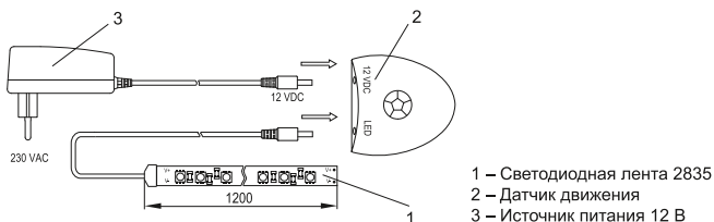
Рисунок 12 – Подключение комплекта LSR1-1-060-20-1-D12-S3
