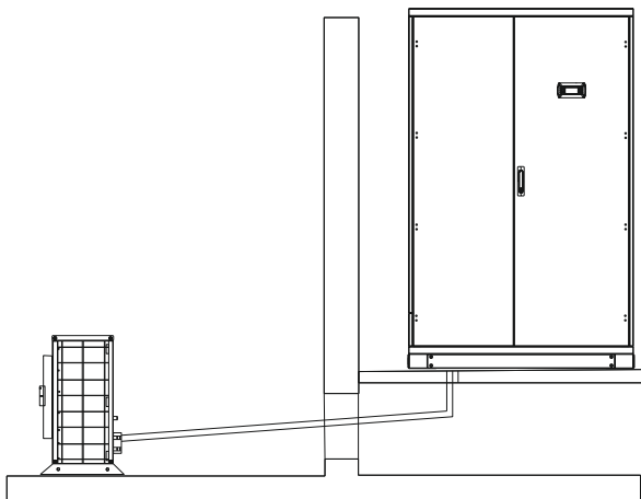
Рисунок 9 – Конденсатор находится на уровне компрессора
