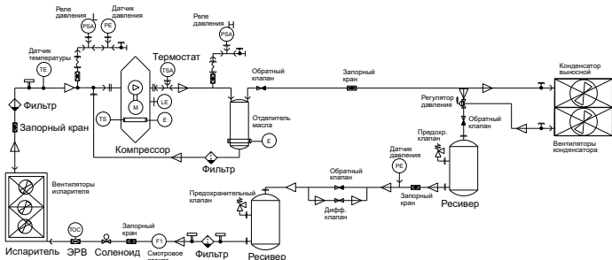
Рисунок 2 – Схема фреоновой промышленного кондиционера
