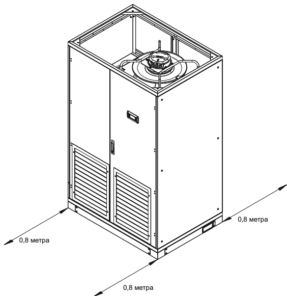
Рисунок 5 – Пример размещения кондиционера
