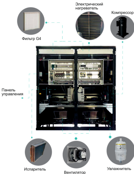
Рисунок 1 – Основные элементы и агрегаты кондиционера
