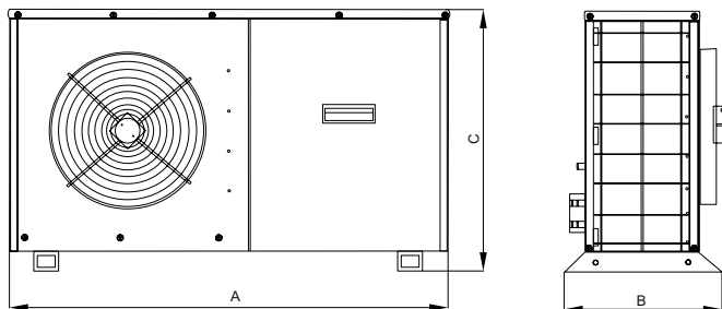
Рисунок 4 – Внешний вид выносного конденсатора для типа AIR CAB
