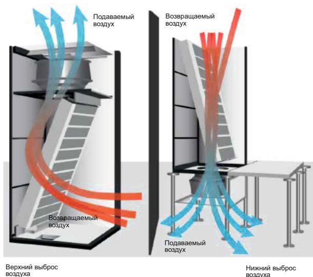
Рисунок 6 – Движение воздуха внутри кондиционера
