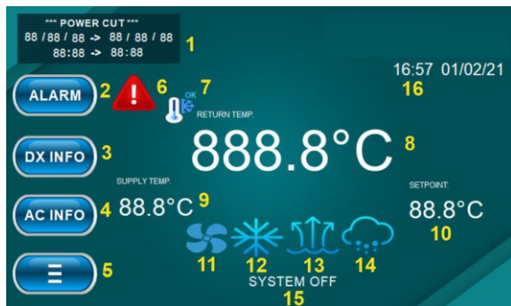
Рисунок 12 – Сенсорная панель управления
