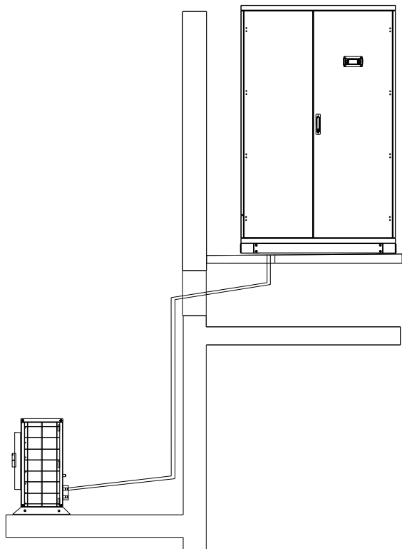
Рисунок 8 – Конденсатор находится ниже компрессора
