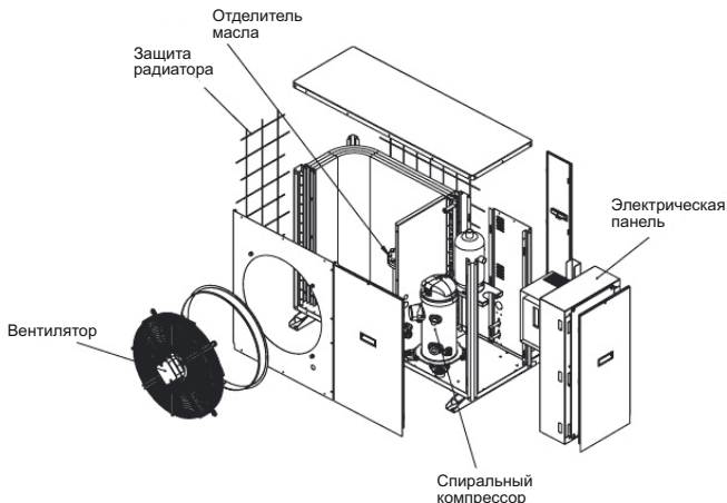
Рисунок 10 – Основные компоненты конденсатора
