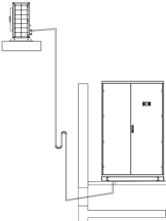
Рисунок 7 – Конденсатор находится выше компрессора
