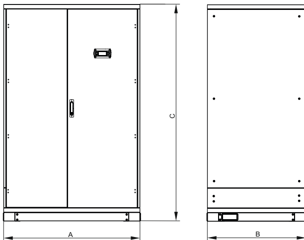
Рисунок 3 – Внешний вид кондиционера типа AIR CAB, FLUID CAB, WATER CAB
