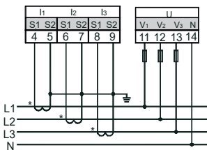
з) Трехфазное, четырехпроводное подключение (3-Ф. 3-ПР., 3-ТТ, 0-ТН)
