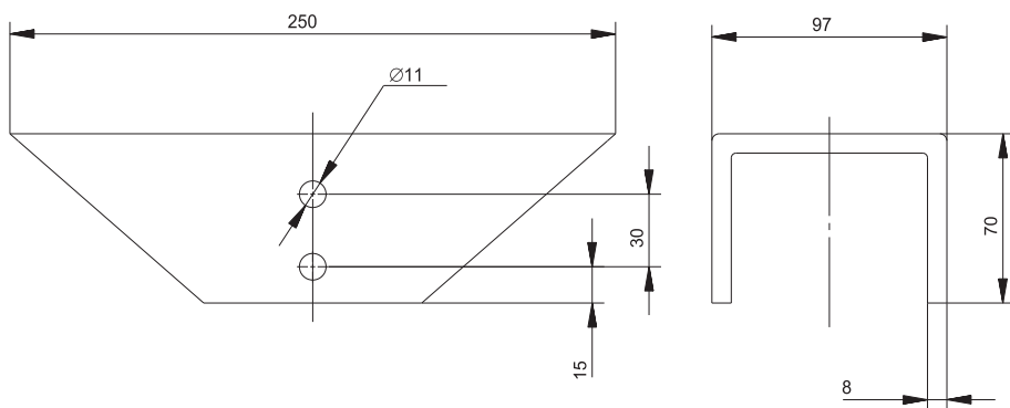
Рисунок / Figure 1 – Крепление потолочное для П-профиля / Ceiling attachment for U-shaped profile
