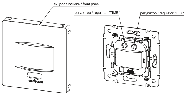
Рисунок 3 – Конструкция датчика движения / Figure 3 – Motion sensor design / 3-сურет – Қимыл датчигінің құрылымы / Figura 3 – Designul senzorului de mișcare / ნახატი 3 – მოძრაობის გადამწოდის კონსტრუქცია / 3-сურет – Қыймыл сенсорунун конструкциясы / Расми 3 – Сохти сенсори ҳаракат / 3-rasm – Harakat sensorining konstruksiyasi
