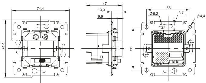
Рисунок 1 – Габаритные и установочные размеры / Figure 1 – Overall and installation dimensions / 1-сურет – Габариттік және орнату өлшемдері / Figura 1 – Dimensiunile generale și de instalare / ნახატი 1 – გაბარიტული და საყენებელი ზომები / 1-сүрөт – Көлөм жана орнотмо өлчөмдөрү / Расми 1 – Андозაи умумий ва насбии / 1-rasm – Umumiy va o'rnatish o'lchamlari
