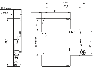
a) Контакт состояния / State contact AR-AUX-SC-240–415
