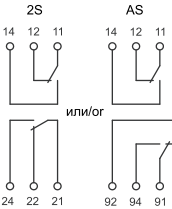
c) Переключаемый контакт / Dual contact AR-AUX-DC-240–415
