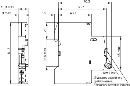
b) Аварийный контакт / Alarm switch AR-AUX-AC-240–415
