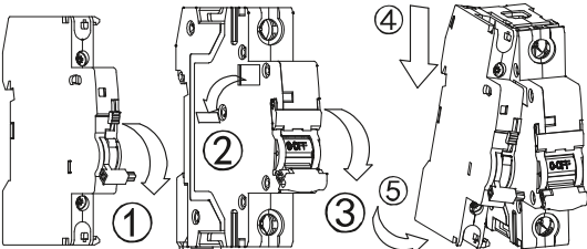
Рисунок 2 – Присоединение контакта к защитному устройству / Figure 2 – Connection of the contact to the protective device
