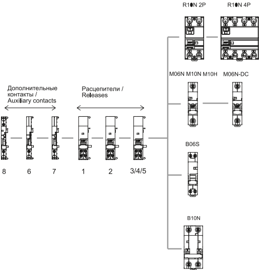
Рисунок 1 – Логика подключения аппаратов защиты и дополнительных устройств серии ARMAT / Figure 1 – Connection logic of protective devices and accessories of ARMAT series
