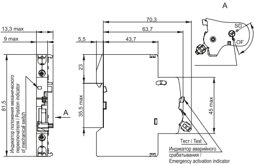
c) Переключаемый контакт / Dual contact AR-AUX-DC-240–415
