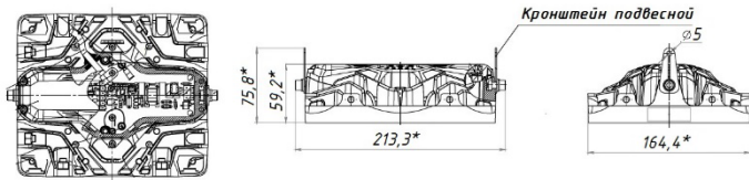
Рисунок 1 Общий вид светильника «L-pixel 1» Подвесное крепление
