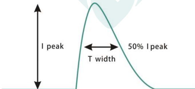
Inrush current(DL-200W-A/P/X-MXG)
