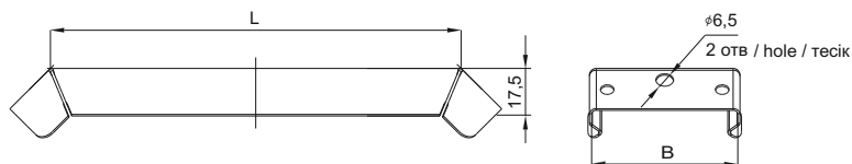
Рисунок 12 – Крышка поворота вертикального внешнего 90 град. / Figure 12 - Cover of 90°vertical external bend / 12 сурет – 90 град. сыртқы вертикалды бұрылыстың қақағы
