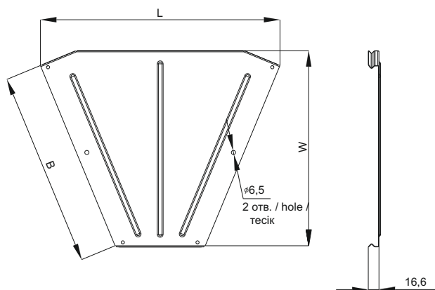
Рисунок 10 – Крышка поворота 45 град. / Figure 10 - Cover of 45° bend / 10 сурет – 45 град. бұрылыстың қаптағы
