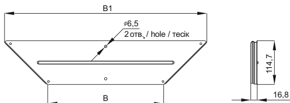
Рисунок 2 – Крышка отвода Т-образного / Figure 2 - T-branch cover / 2 сурет - Т-тәріздес бұрманың қақпағы
