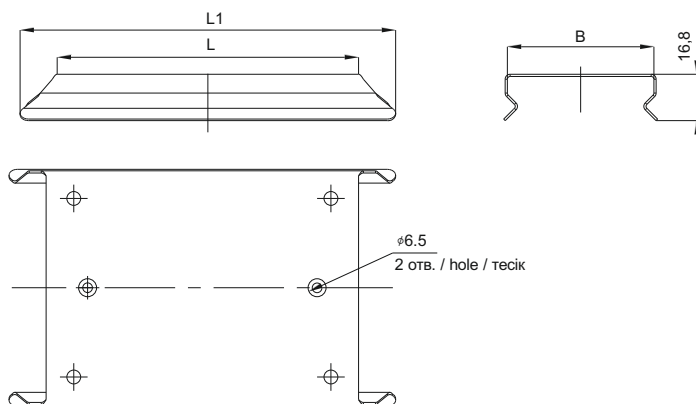
Рисунок 14 – Крышка поворота вертикального внутреннего 90 град. / Figure 14 - Cover of 90°vertical internal bend / 14 сурет – 90 град. ішкі вертикалды бұрылыстың қақағы
