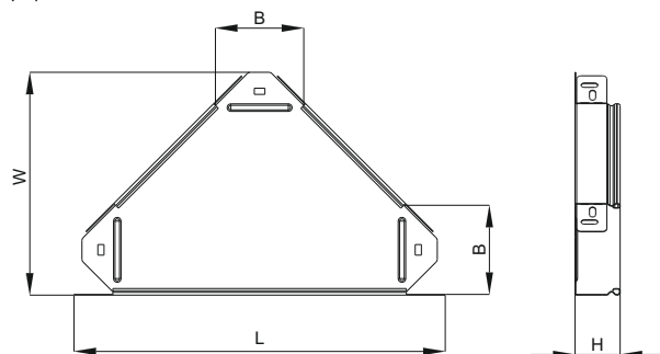
Рисунок 4 – Крышка крестовины / Figure 4 - Cover of the crossover / 4 сурет - Айқастырманың қақпағы
