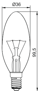
Рисунок 2. Лампа C35 цоколь E14
