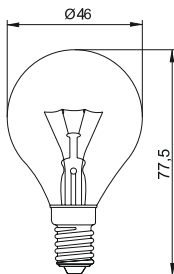
Рисунок 4. Лампа G45 цоколь E14
