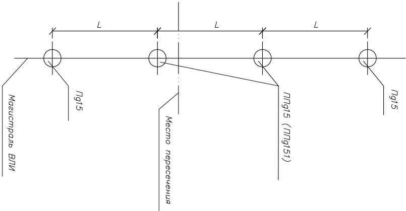
Схема установки опоры на ВЛИ
