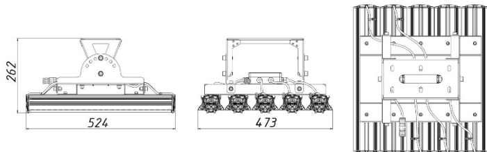
Рисунок 2 Светильник «L-industry Turbine HB5»
