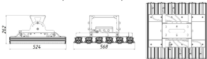
Рисунок 3 Светильник «L-industry Turbine HB6»
