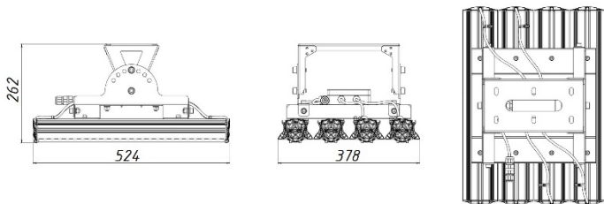
Рисунок 1 Светильник «L-industry Turbine HB4»
