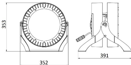
Рисунок 1 Общий вид светильника L-industry II banner Pro.
