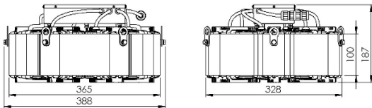
Рисунок 1 Общий вид светильника «L-lego II 330» Подвесное крепление
