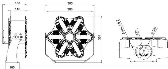
Рисунок 2 Общий вид светильника «L-lego II 330 banner» Поворотное крепление
