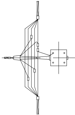
Схема ответвления к вводу в здания в одну сторону 4х жил СИП
