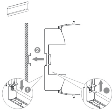
Рисунок 2 – Монтаж модуля на Т-образную монтажную рейку
