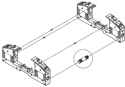
Рисунок 1 – Монтаж модулей между собой
