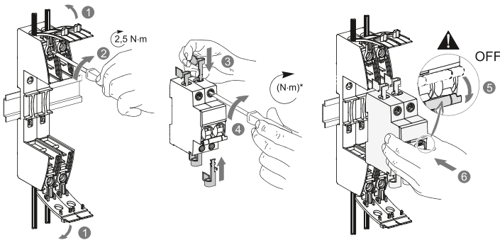
Рисунок 4 – Монтаж автоматического выключателя
