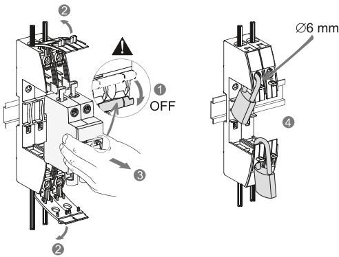
Рисунок 5 – Демонтаж автоматического выключателя
