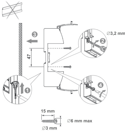
Рисунок 3 – Монтаж модуля на монтажную панель
