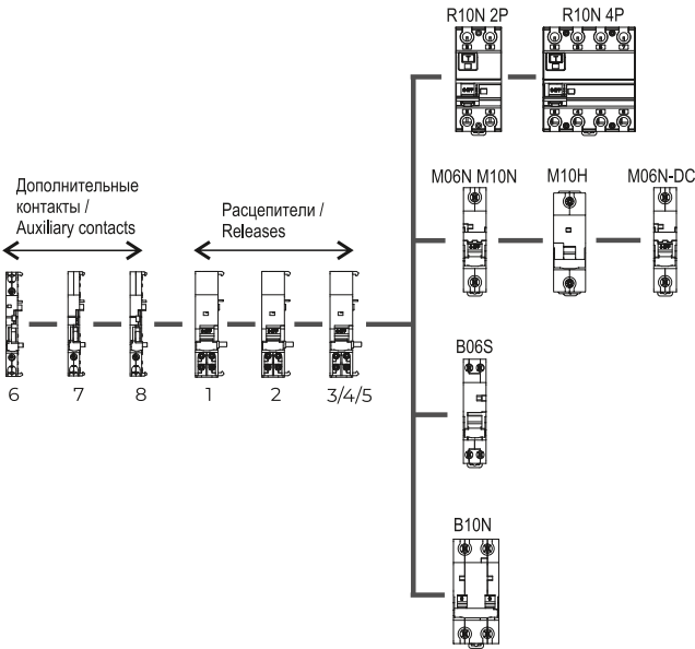
Рисунок 1 – Логика подключения аппаратов защиты и дополнительных устройств серии ARMAT/ Figure 1 – Connection logic of ARMAT series protection devices and accessories
