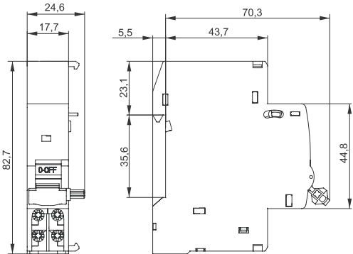
Габаритные и установочные размеры расцепителя / Overall and mounting dimensions of release
