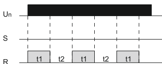
Рисунок 3 – Функциональная диаграмма циклического реле с циклом, начинающимся с импульса (без перемычки между контактами S и A1) / Figure 3 – Functional diagram of periodic relay with a cycle, starting with a pulse (without jumper between contacts S and A1) / 3 сурет – Импульстен басталатын циклді циклдік реленің функционалдық диаграммасы (S және A1 түйіспелерінің арасында жалғастырғышсыз)
