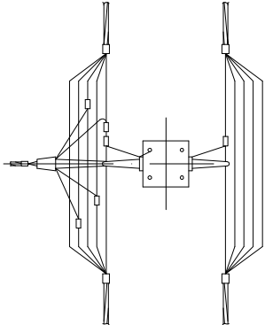
Схема ответвления к вводу в здания в одну сторону 4х жил СИП
