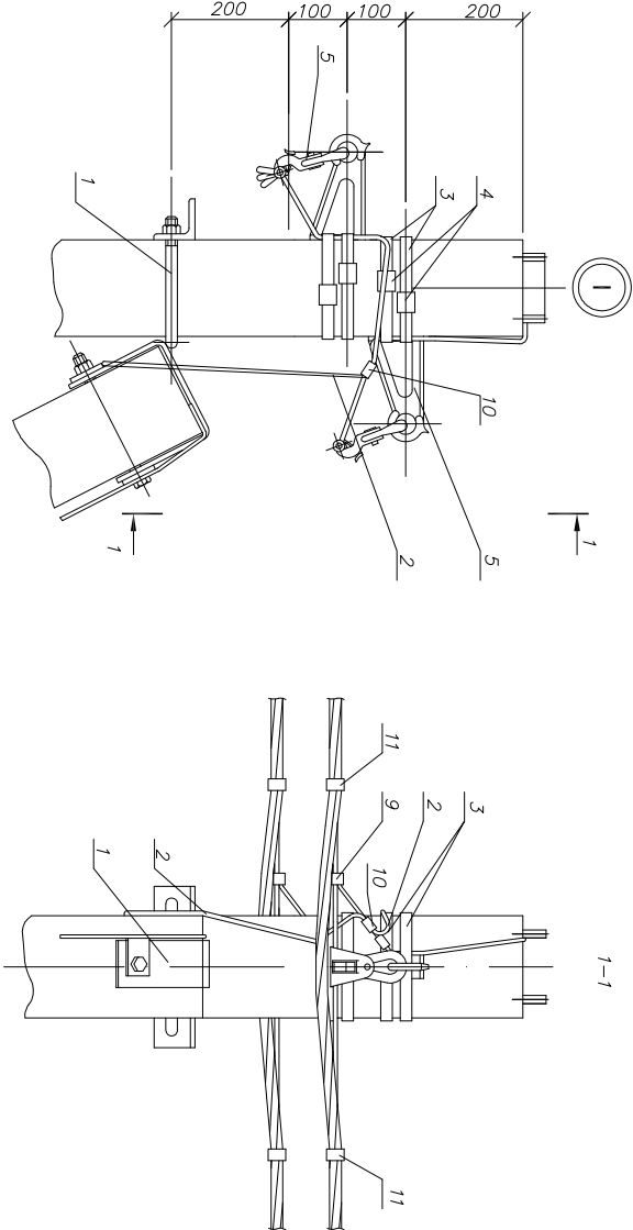
Отделение к вводу в здания в одну сторону от ВЛ проводов СИП
