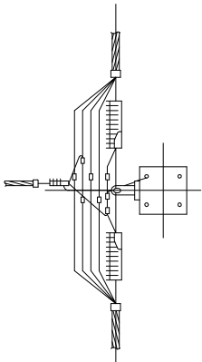
Схема ответвления к входу в здания в одну сторону в жил СИП
