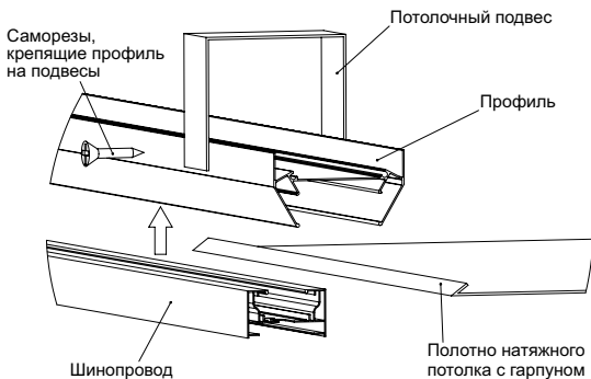
Рисунок 4 – Схема установки профиля
