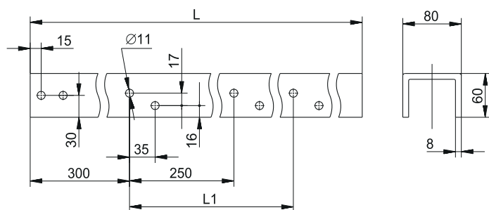
Рисунок / Figure 2 – Профиль П-образный перфорированный по высоте 80×60 мм / Heightwise perforated U-shaped profile 80×60 mm
