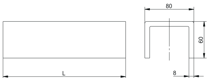
Рисунок / Figure 4 – Профиль П-образный неперфорированный 80×60 мм / Non-perforated U-shaped profile 80×60 mm
