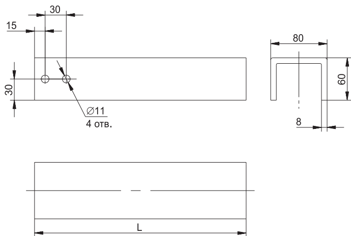
Рисунок / Figure 1 – Профиль П-образный перфорированный 80×60 мм / Perforated U-shaped profile 80×60 mm
