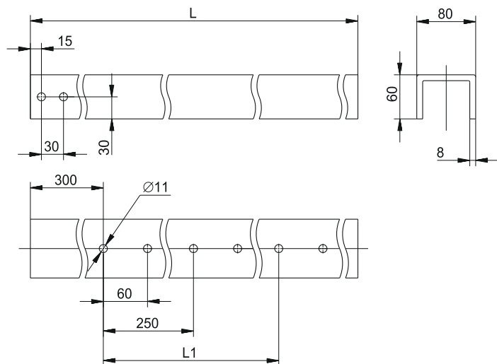
Рисунок 3 – Профиль П-образный перфорированный по ширине 80×60 мм / Breadthwise perforated U-shaped profile 80×60 mm
