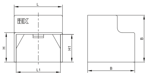
Рисунок 2 – Угол Т-образный KMT / Figure 2 – T-bend KMT / 2-сурет – Т-терізді бұрыш KMT
