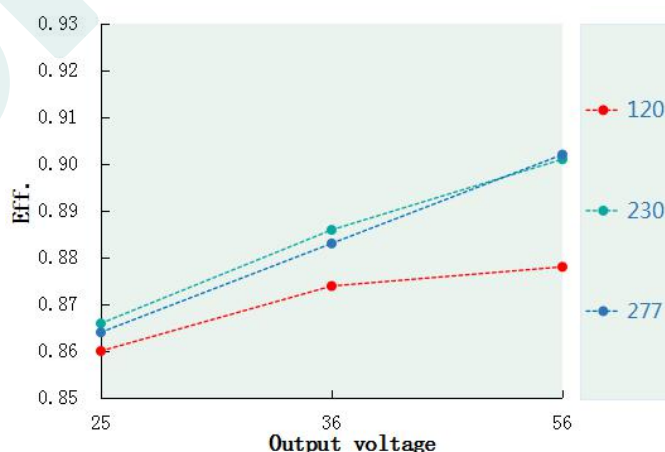
Eff. VS Output voltage(DL-100W-V56A/P/X-MXG)
