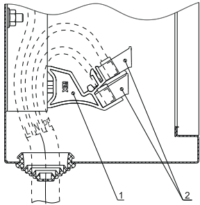
1 – стойка для суппортов / support pillar / суппорттар сересі 2 – суппорты для шин N/PE / holders for N/PE busbars / N/PE шиналардағы суппорттар
