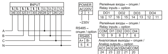
а) схема подключения мультиметра LCD к четырехпроводной сети при I \leq 5 A, U \leq 600 В / LCD multimeter connection diagram to a four-wire network at I \leq 5 A, U \leq 600 V
