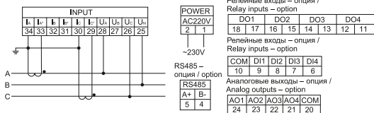
д) схема подключения мультиметра LCD к трехпроводной сети при I > 5 A, U \leq 600 В / wiring diagram of the multimeter LED, LCD to a three-wire network at I > 5 A, U \leq 600 V
