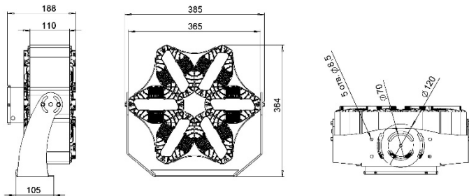
Рисунок 2 Общий вид светильника «L-lego II 330 banner» Поворотное крепление
