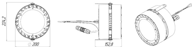
Рисунок 1 Общий вид светильника L-industry II .
