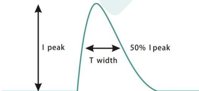
Inrush Current(DL-50W-A/P/X-MXG)
