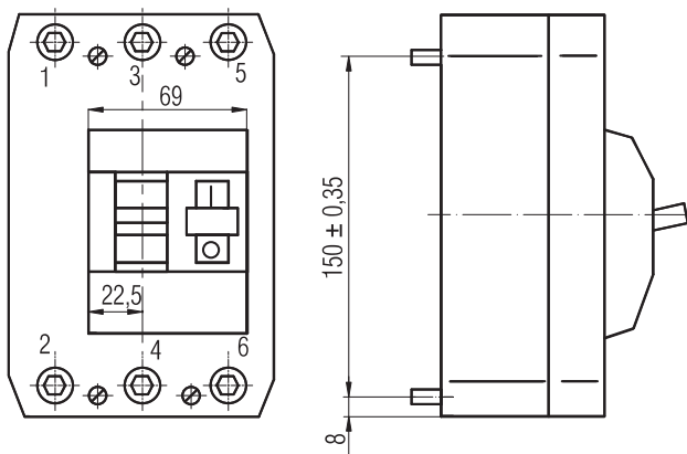
Рисунок А.2 - Габаритные и установочные размеры выключателя типа BA06-36.
