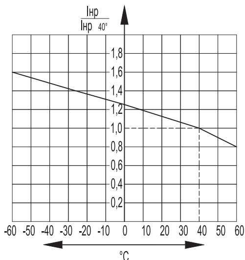
Рисунок Г.1 - Зависимость номинального тока выключателя (расцепителя), выраженного в кратностях к номинальному току при 40 ^\circ\text{C} , от температуры окружающего воздуха (для выключателей исполнения УХЛЗ).
