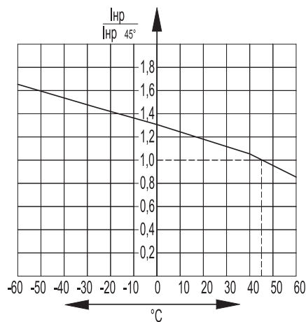
Рисунок Г.2 - Зависимость номинального тока выключателя (расцепителя), выраженного в кратностях к номинальному току при 45 ^\circ\text{C} , от температуры окружающего воздуха (для выключателей исполнения ТЗ).
