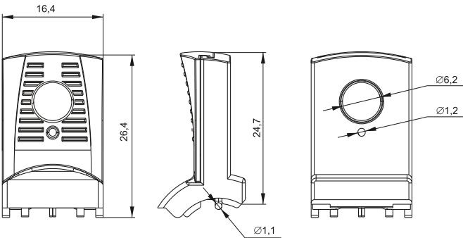
Рисунок 1 – Габаритные размеры блокировки / Figure 1 – Overall dimensions of the interlock
