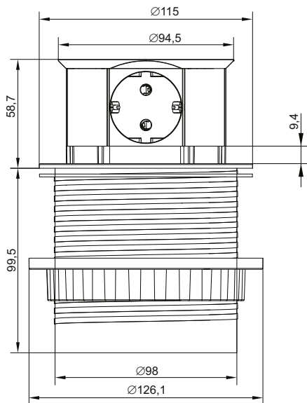
Удлинитель U03 Qi / Cord extention set U03 Qi / Ұзартқышы U03 Qi
