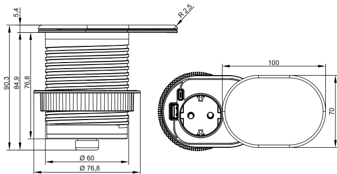
Удлинитель У01 / Cord extension set U01 / Ұзартқышы У01
