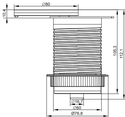
Удлинитель У01Qi / Cord extension set U01Qi / Ұзартқышы У01Qi
